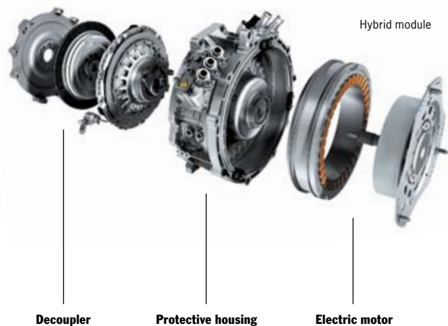
Decoupler
